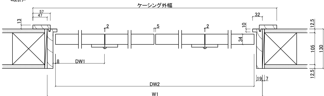
ヨコ断面
