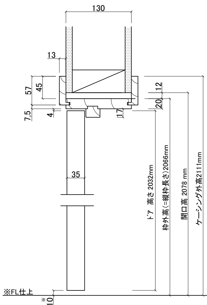
タテ断面
