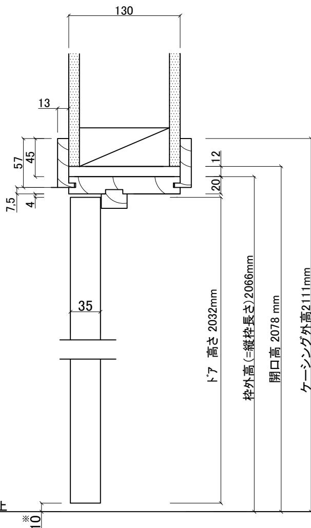
調整丁番仕様(親親)
